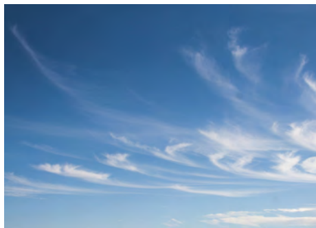
Cirrus
