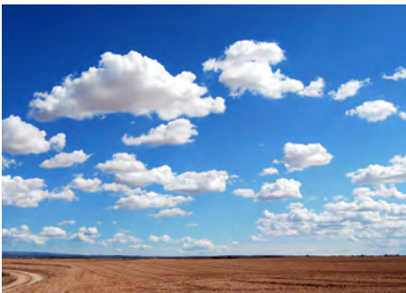
Cumulus
