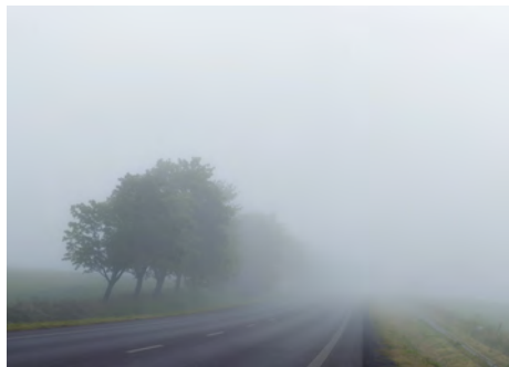
Fog
